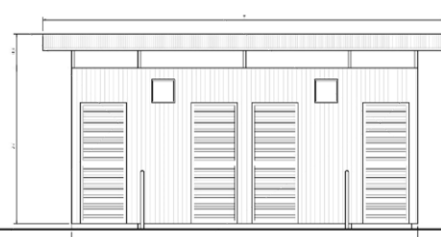
VISTA FRENTE 2 MÓDULOS ACESSÍVEIS / 2 MÓDULOS COMUNS
