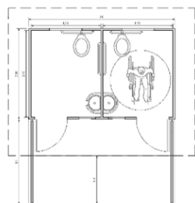
SANITÁRIOS - PLANTA BAIXA 2 MÓDULOS ACESSÍVEIS
