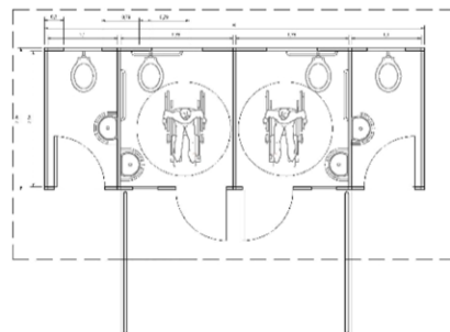
SANITÁRIOS - PLANTA BAIXA 2 MÓDULOS ACESSÍVEIS / 2 MÓDULOS COMUNS
